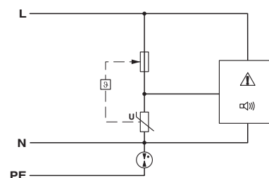
Kapcsolási rajz
