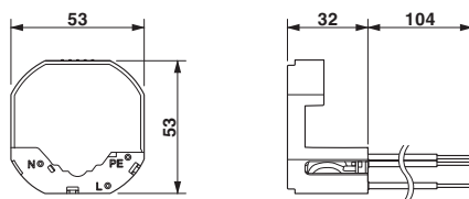
Méretrajz
